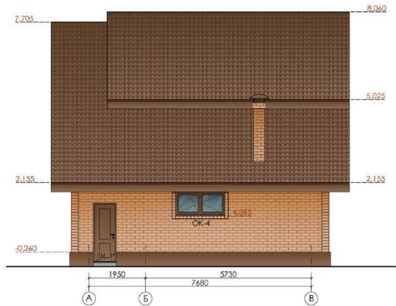
Фасад в осях А-В
