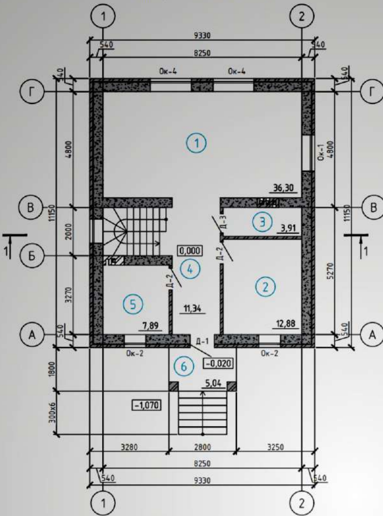
План первого этажа на отм. 0,000
